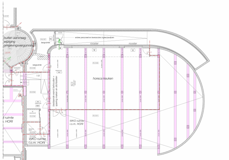
LAAG-2 nieuw
