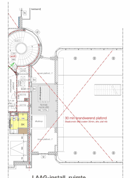
LAAG-install. ruimte
