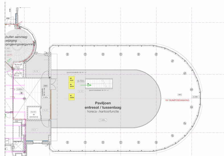
LAAG-entresol nieuw
